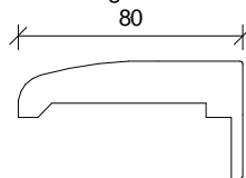
Bekleidung FB bombiert
