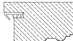
ABZ-LH Rahmenverbindung auf Gehrung
