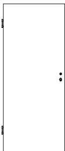
VN/K3 (Klima* 3) mit Alueinlage, Falzdichtung, Schall-Ex Türstärke 47
