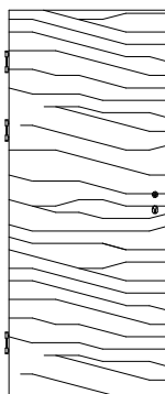
FN/Q3 querfurniert (Klima 3) Türstärke 43 mm, PZ, Schalllex
