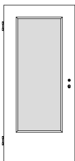
LN/K2-LA 1 mit Alueinlage
