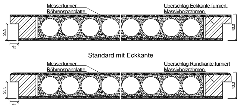
Modell RI/D1 + RI/X1 wahlweise mit Rundkante
