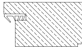
ABZ-INL Rahmenverbindung auf Gehrung
