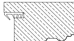
ABZ-LH Rahmenverbindung auf Gehring
